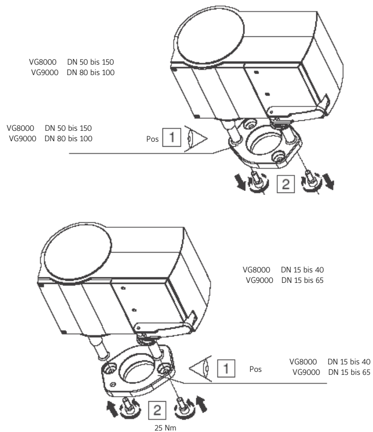
Abbildung 5: Montage des Antriebs VA1000 in Abhängigkeit von der Ventillinnenweite
