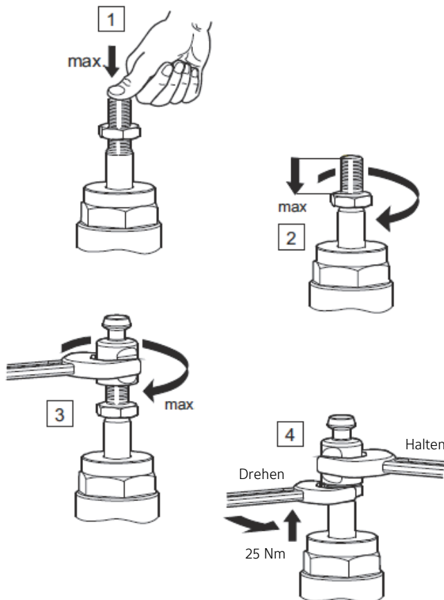
Abbildung 37: Montage des Adapterkits VA1000-ITT-KITx (Teil 1 von 3)
