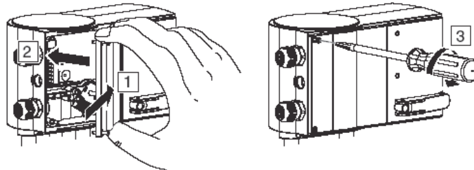
Abbildung 35: Montage VA1000-P2 (Teil 6 von 6)
