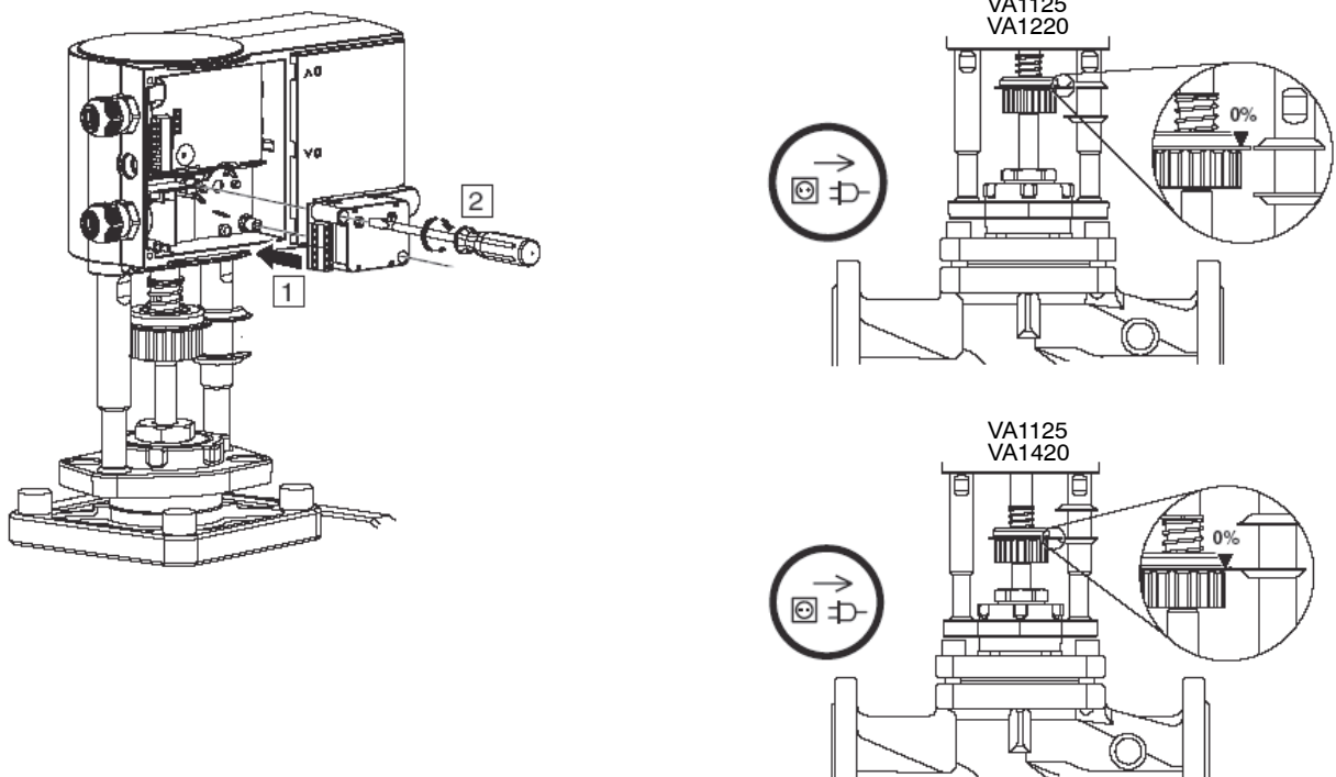
Abbildung 22: Montage VA1000-S2 (Teil 2 von 4)
