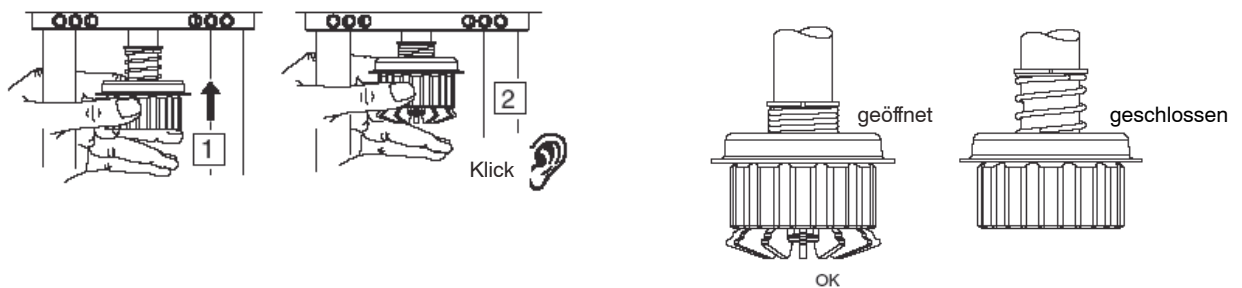
Abbildung 2: Funktionsweise des Ventilanschlusses
