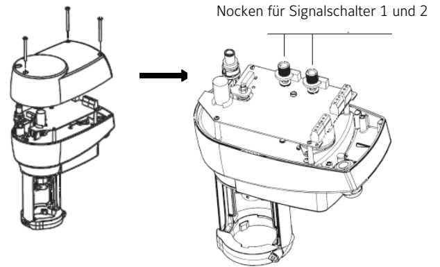
Abbildung 4: Einstellen der Signalschalter durch Einstellen der Nocken (modellabhängig)
