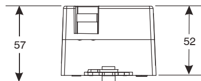
Abbildung 1: Abmessungen (mm) M9102 und M9104
