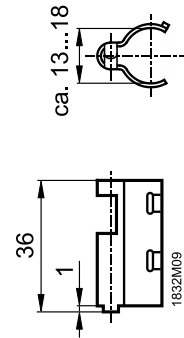
Changeover- Bausatz ARG22.1 für Rohranlege- montage
