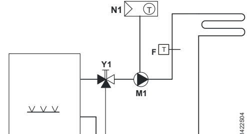
Raumthermostat mit direkter Ansteuerung einer wasserbasierten Fussbodenheizung
