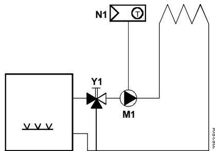
Umwälzpumpe mit Vorregelung durch Handmischer
