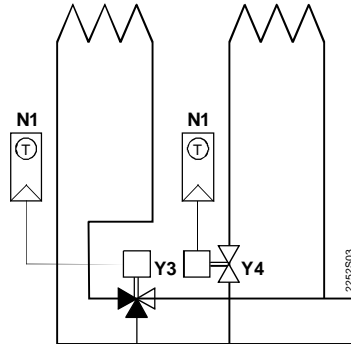
Zonenventil
